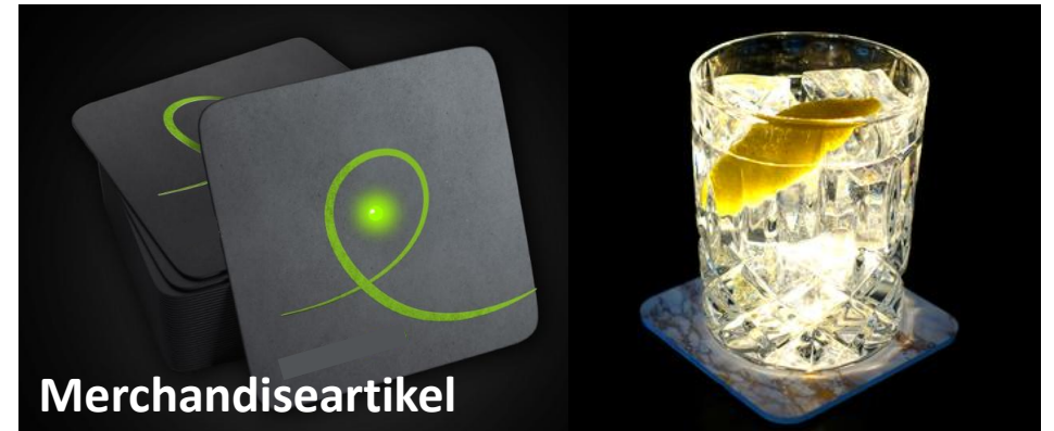
Interagierende NFC-Technologien
